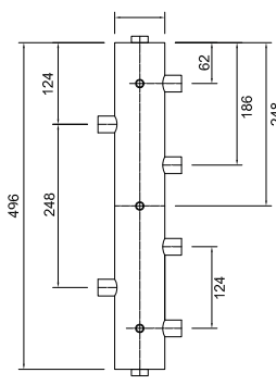
COD. ACC740C002 Separador Hidráulico 5", 4VX2" + 2VX3/4", Aislación
