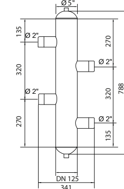
COD. ACC740C002 Separador Hidráulico 5", 4VX2" + 2VX3/4", Aislación
