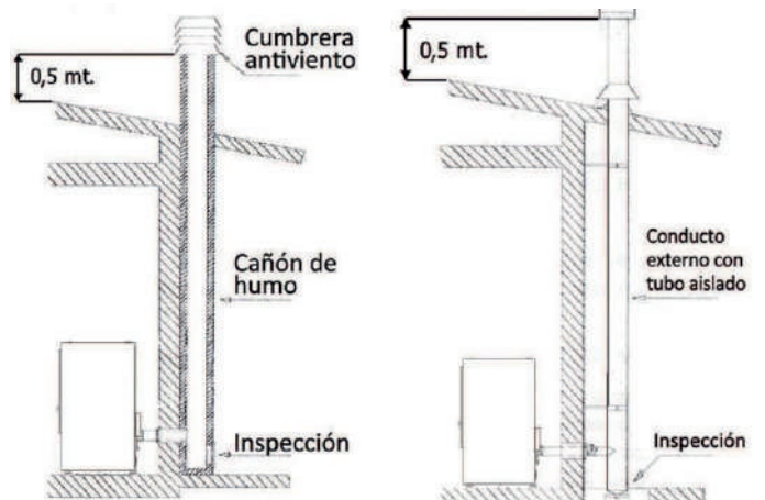
Fig. 3 : conexión a un conducto externo con tubo aislado o doble pared una cumbrera antiviento.
