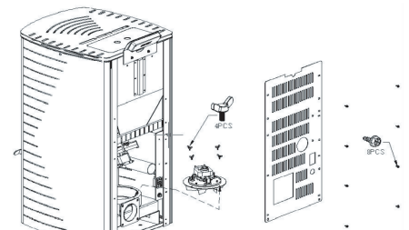
Como reemplazar el ventilador de combustión
