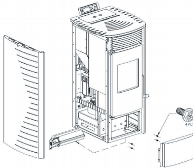
Como reemplazar el ventilador de habitación (soplador)
